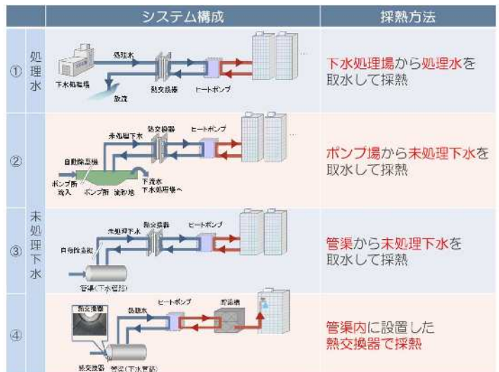
図2 下水熱利用システムの主な構成
